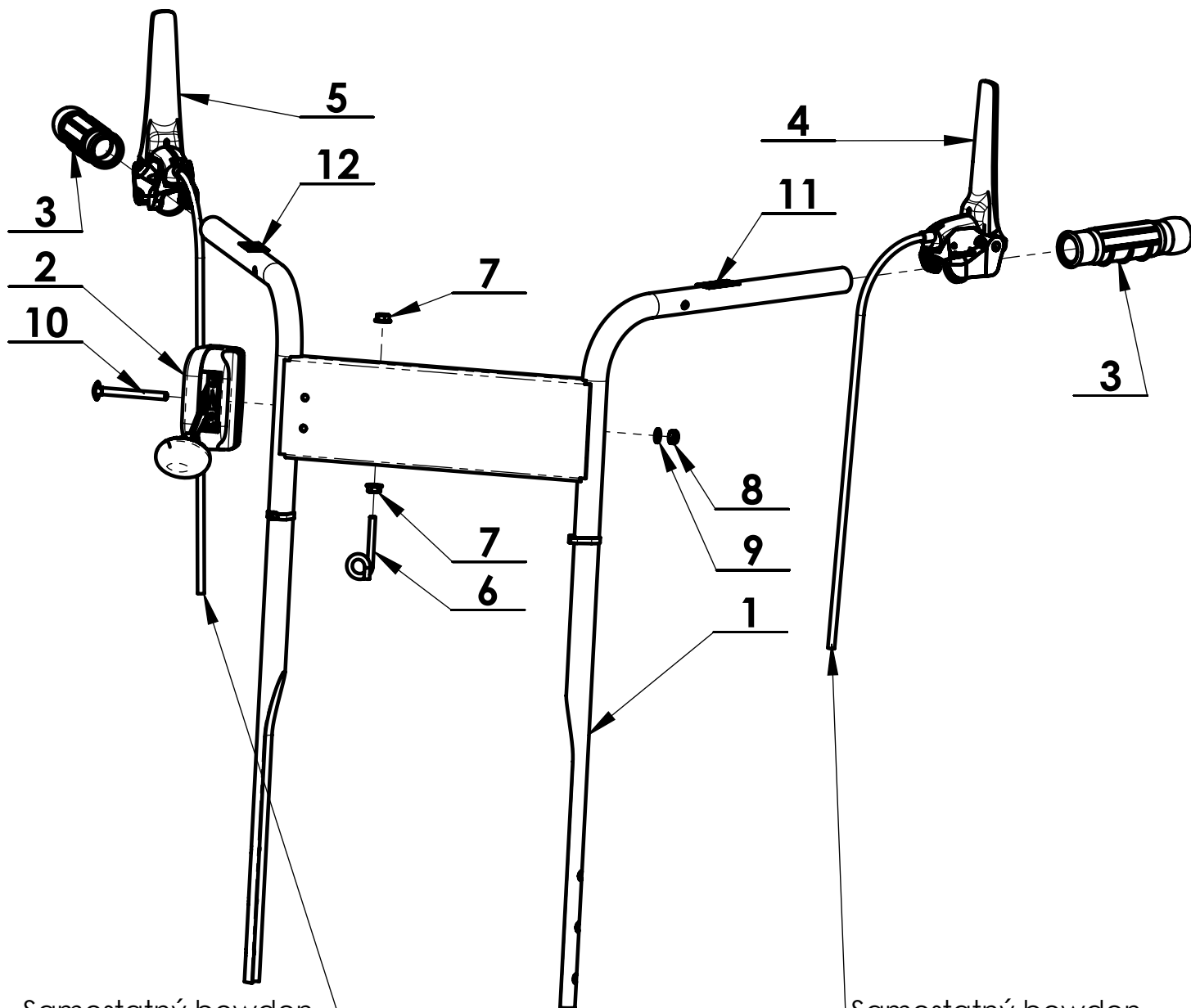
Samostatný bowden kladky pohonu obj. č. 2006100045
