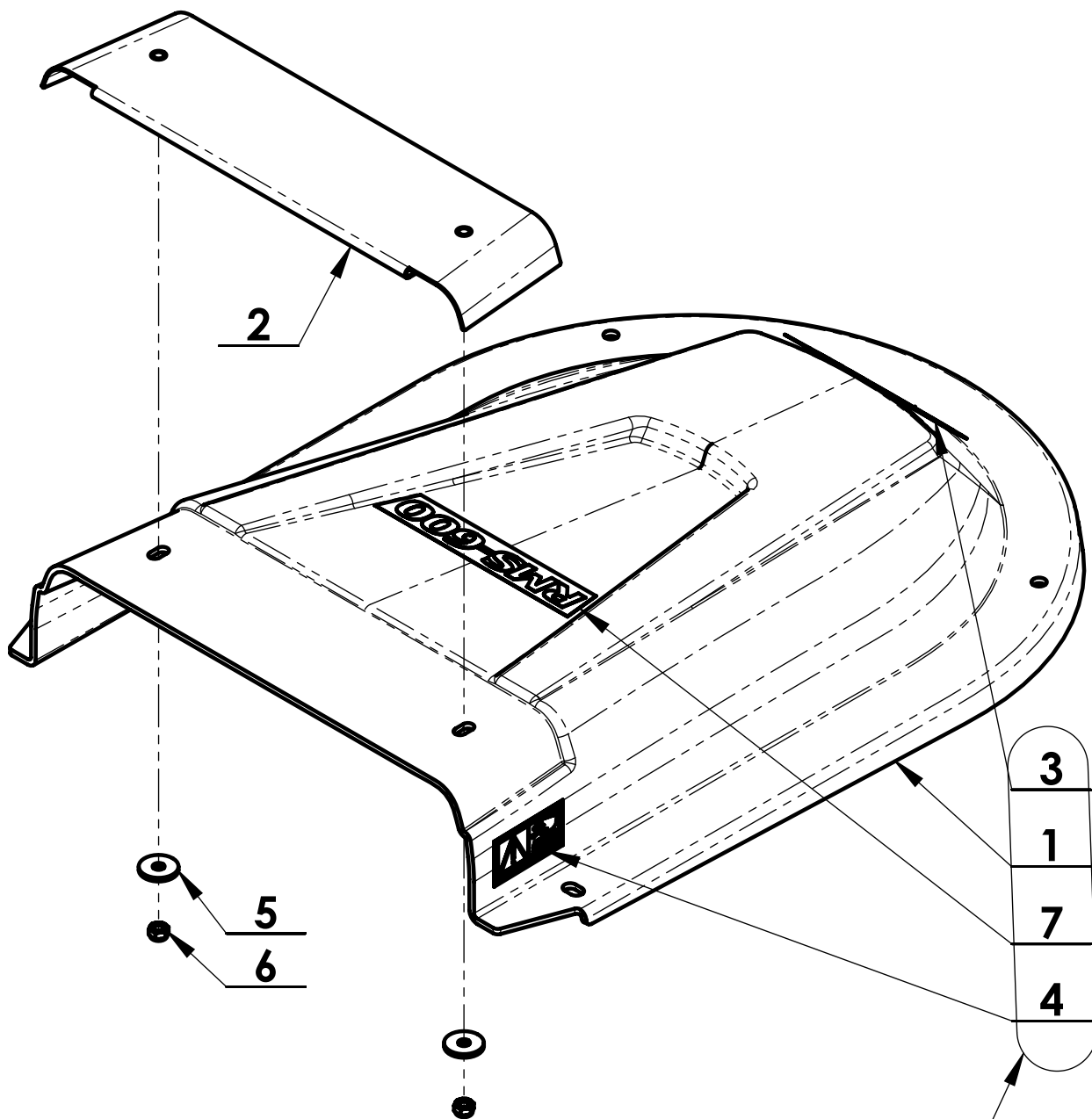
Kryt řemene RAPTOR poz. 1 sestava pro náhradní díly objednáací číslo 3005900045
